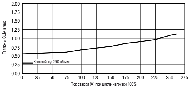
Кривая потребления топлива (дизель)
